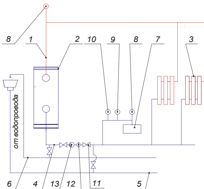
1-главный стояк;2-котел;3-радиатор;4-трубопровод обратной воды;5-сливная магистраль;6-подпиточный водопровод;7-мембранный расширительный бак;8-автоматический клапан выпуска воздуха;9-манометр;10-предохранительный клапан 300кПа(3,0 кгс/см 2 ); 11-кран;12-фильтр;13-насос.
